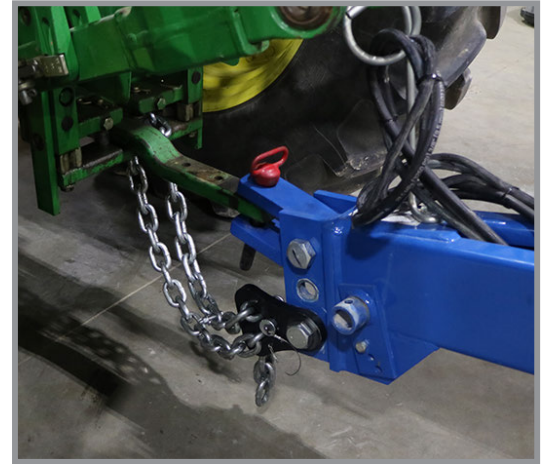
З'єднання тягового бруса і запобіжного ланцюга
