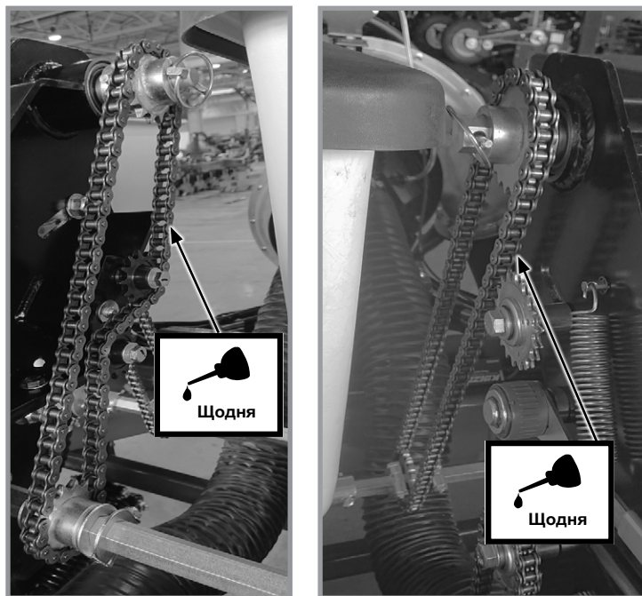
Ланцюг приводу подачі сухих добрив (з обох боків вузла)
