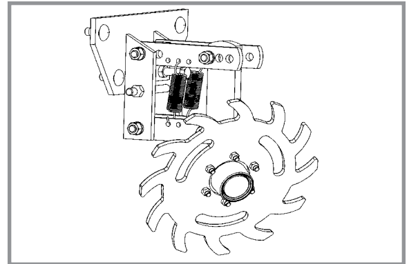
Колеса для пожнивних залишків з кріпленням на висівній секції
