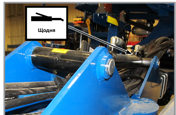
6. Циліндр притиску крила, по 2 на сівалку, по 2 точки змащування на циліндр (по одній на кожному кінці)
