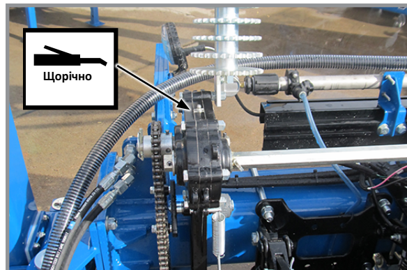
12. Трансмісія
