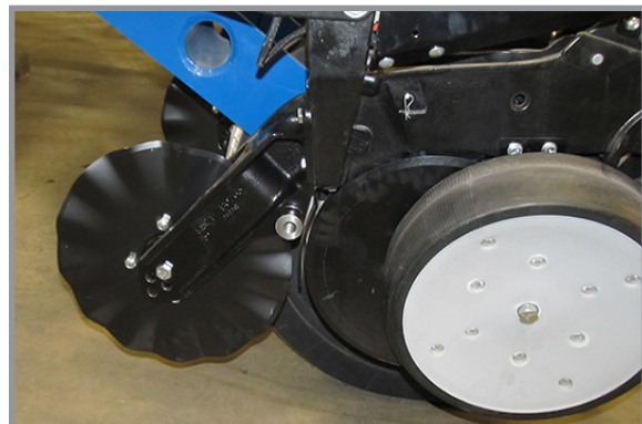
Дискові ножі для нульової обробки ґрунту, що встановлюються на висівні секції
