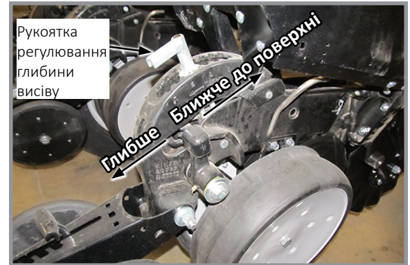
Регулювання глибини висіву
