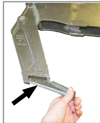
Захист насінняпроводу/внутрішній чистик (Копіююче колесо/дисковий ніж сошника для внесення насіння знятий для більшої наочності)
