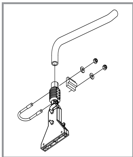
4 ½-дюймова (~12 см) зв'язка з компенсацією нахилу
