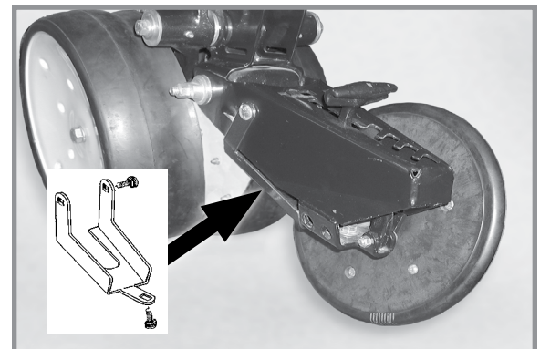
Щиток зашпаровуючого колеса (одне з коліс знято)
