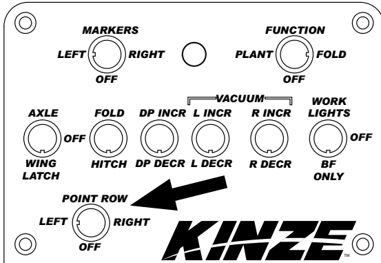
Пульт управління
