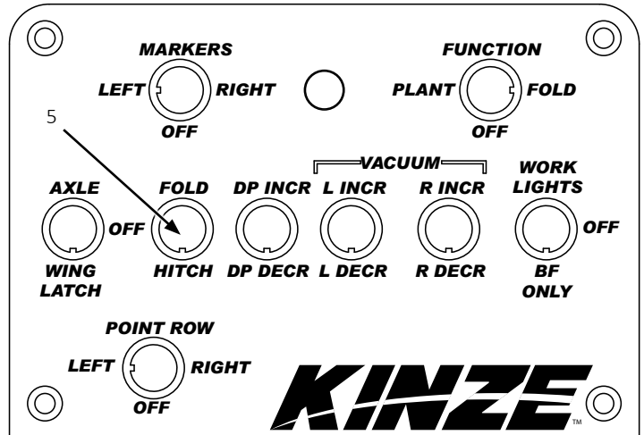
Пульт управління
