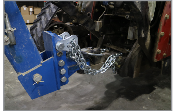
Приєднання запобіжного ланцюга до трактору в разі використання тягового бруса
