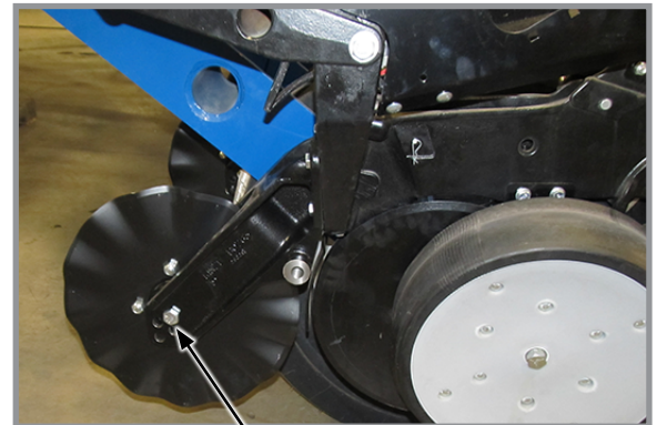
Отвори для регулювання ножів
