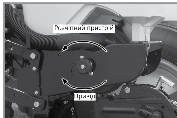
Розчпний пристрій приводу для гранульованих хімікатів
