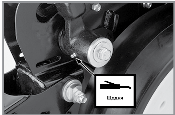
10. Важелі копіюючих коліс - по 1 на важіль
