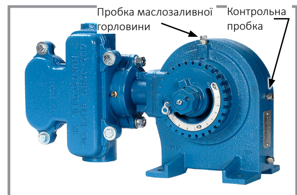
Розташування заливної та контрольної пробки поршневого насоса
