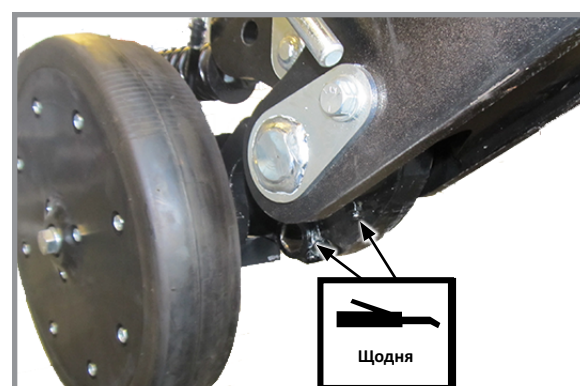
Мастило для очищення - 2 фітінги
