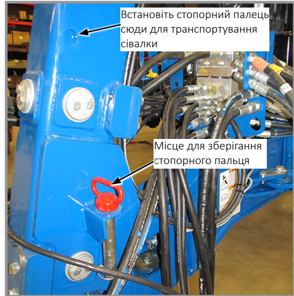
Стопорний палець зчипки дишла
