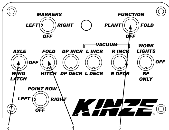
Пульт управління
