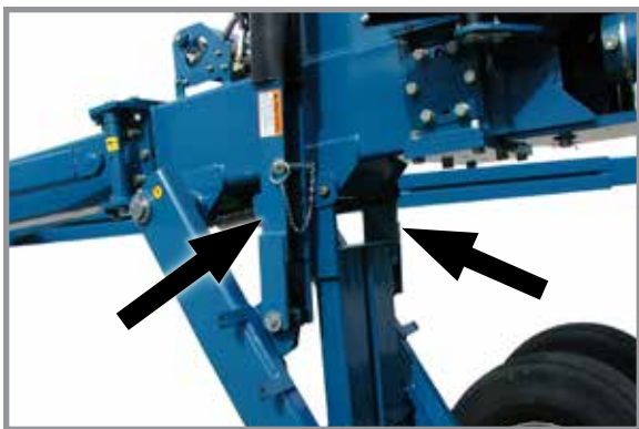
Блокировочные устройства в положении для транспортировки
