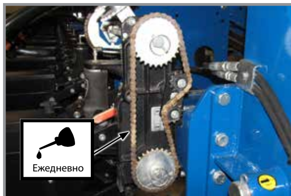
Цепи трансмиссии
