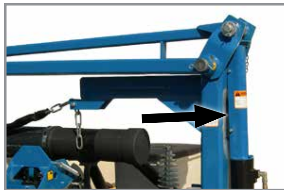
Установленное блокировочное устройство маркера
