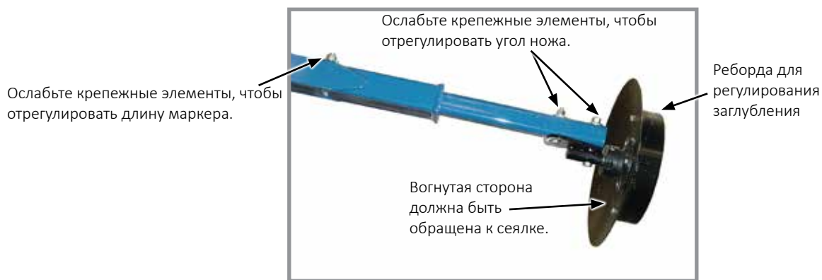
Регулировка угла дискового ножа маркера
