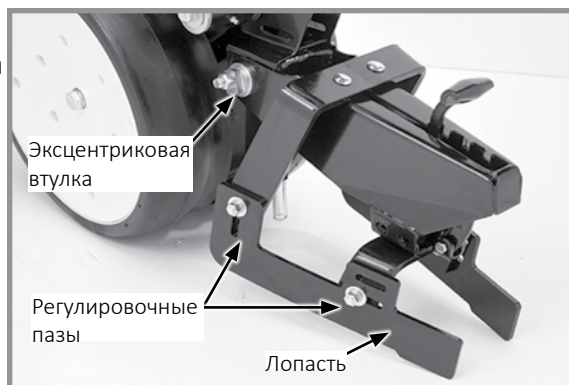
Заделывающее приспособление
