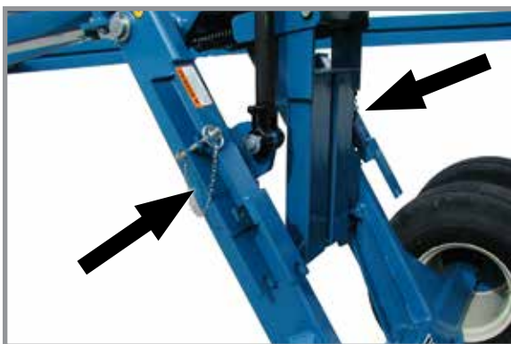
Блокировочное устройство в положении для хранения
