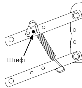
Положение 4 (наибольшее)
