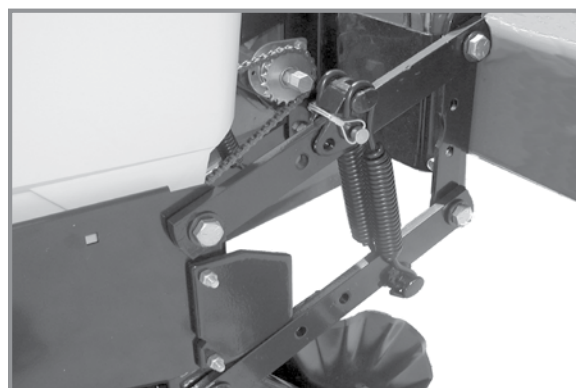
Четыре пружины на ряд (четверенные пружины)
