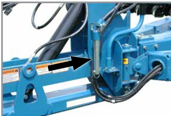
Блокировочное устройство параллелограммных тяг дышла в положении для хранения
